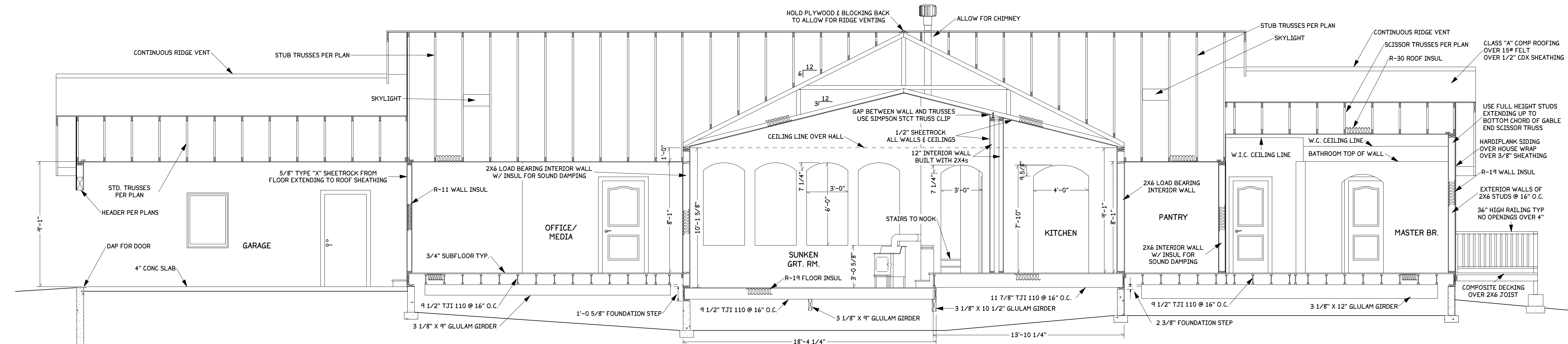
SECTION C-C SCALE: 1/4" = 1'
