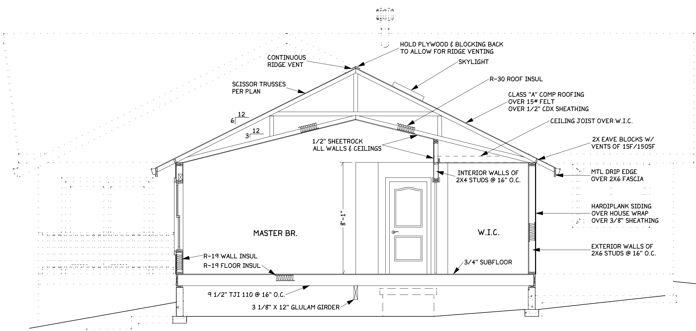
SECTION A-A SCALE: 1/4" = 1'
