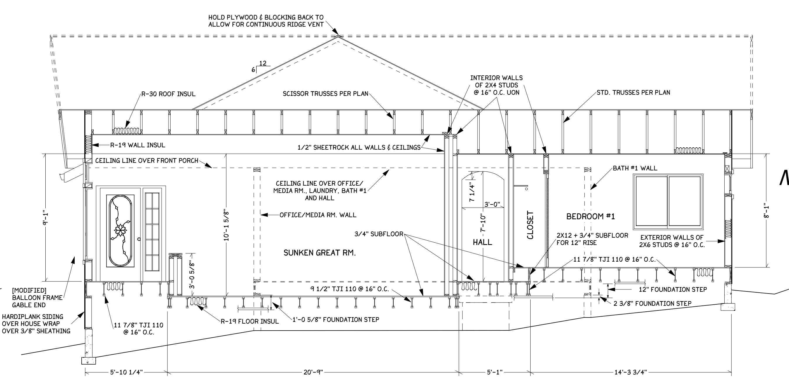
SECTION B-B SCALE: 1/4" = 1'
